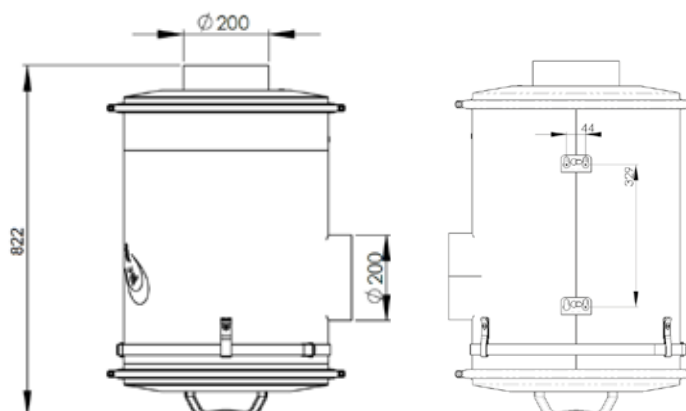
Kontamineringsfritt filterbyte
