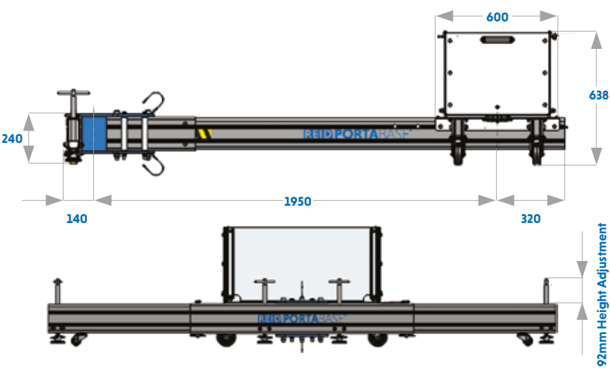
Dimensions
