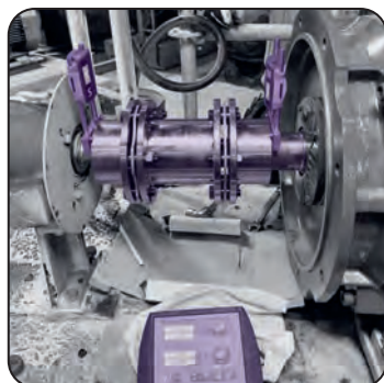
Laser alignment Laseruppriktning Laserlinjauslaitteet Laseropretning Laseroppretting
