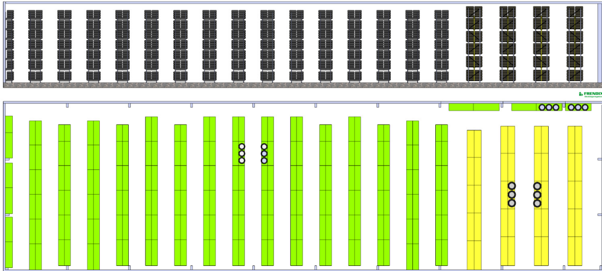
Frendix Däcklagarsystem.Fasta hyllor. Kapacitet PB 7 nivåer (gröna) 3920 satser, max diameter 650mm. Kapacitet SUV 6 nivåer (gula) 720 satser, max diameter 800mm. Totalt 4640 satser (18560 däck). 2012-11-20.
