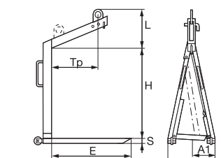
6040-6042 Självbalanserande – hopfällbara gafflar
