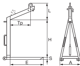
6020-6023 Självbalanserande – fasta gafflar
