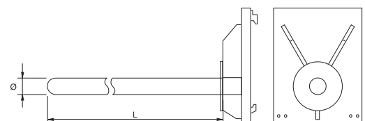
6030-6031 Självbalanserande – ställbara gafflar
