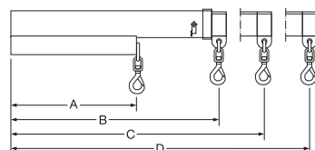
FJCS 45 Kort modell
