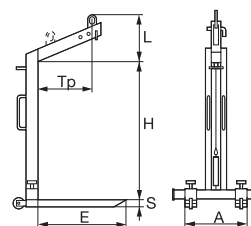
6030-6031 Självbalanserande – ställbara gafflar
