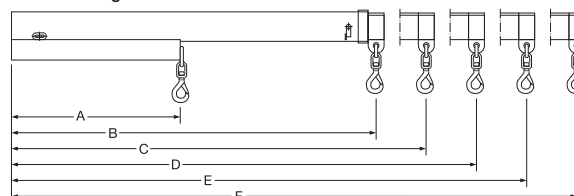
FJCL 45 Lång modell
