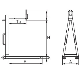
6010-6011 Manuellt flyttbar lyftögla – fasta gafflar
