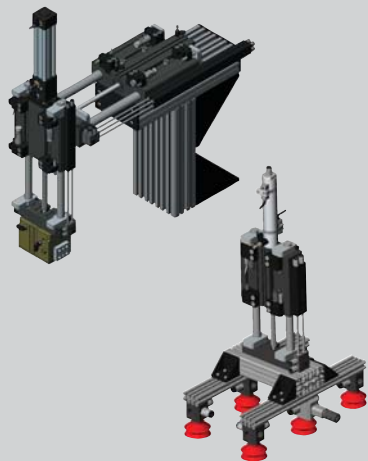
DIRECTCONNECT™ Plockmoduler
