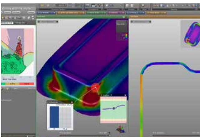
Simuleringstester med AutoForms programvara.
