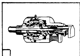
DEUBLIN Kopplingar / ångboxar
